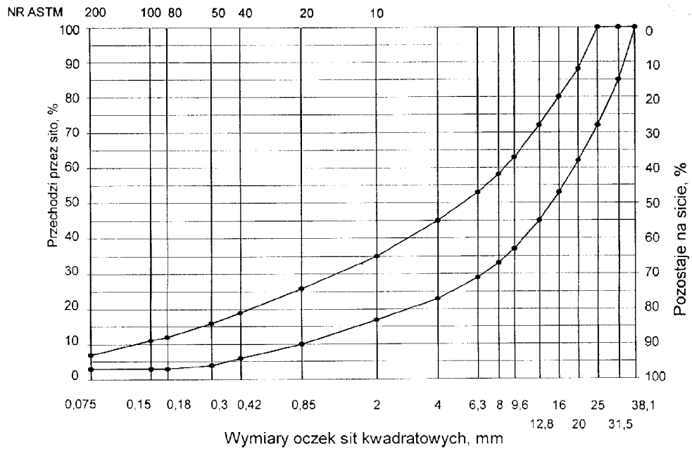
Rys.1. Krzywe graniczne uziarnienia mieszanek mineralnej BA od 0 do 31,5 mm do podbudowy nawierzchni drogi o obciążeniu ruchem KR 1 lub KR 2
