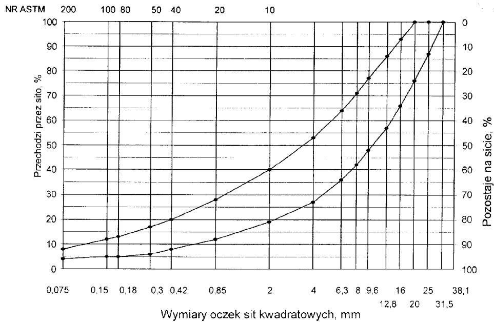
Rys.2. Krzywe graniczne uziarnienia mieszanek mineralnej BA od 0 do 25mm do podbudowy nawierzchni drogi o obciążeniu ruchem KR 1 lub KR 2
