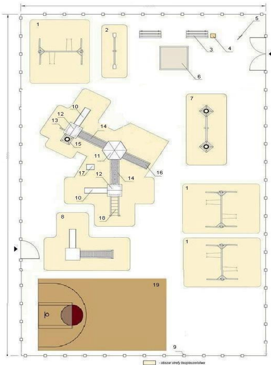
PLAC ZABAW plan sytuacyjny ZESTAW 3 + BOSIKO
